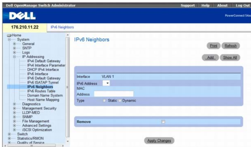
図 6-39. IPv6 近隣
